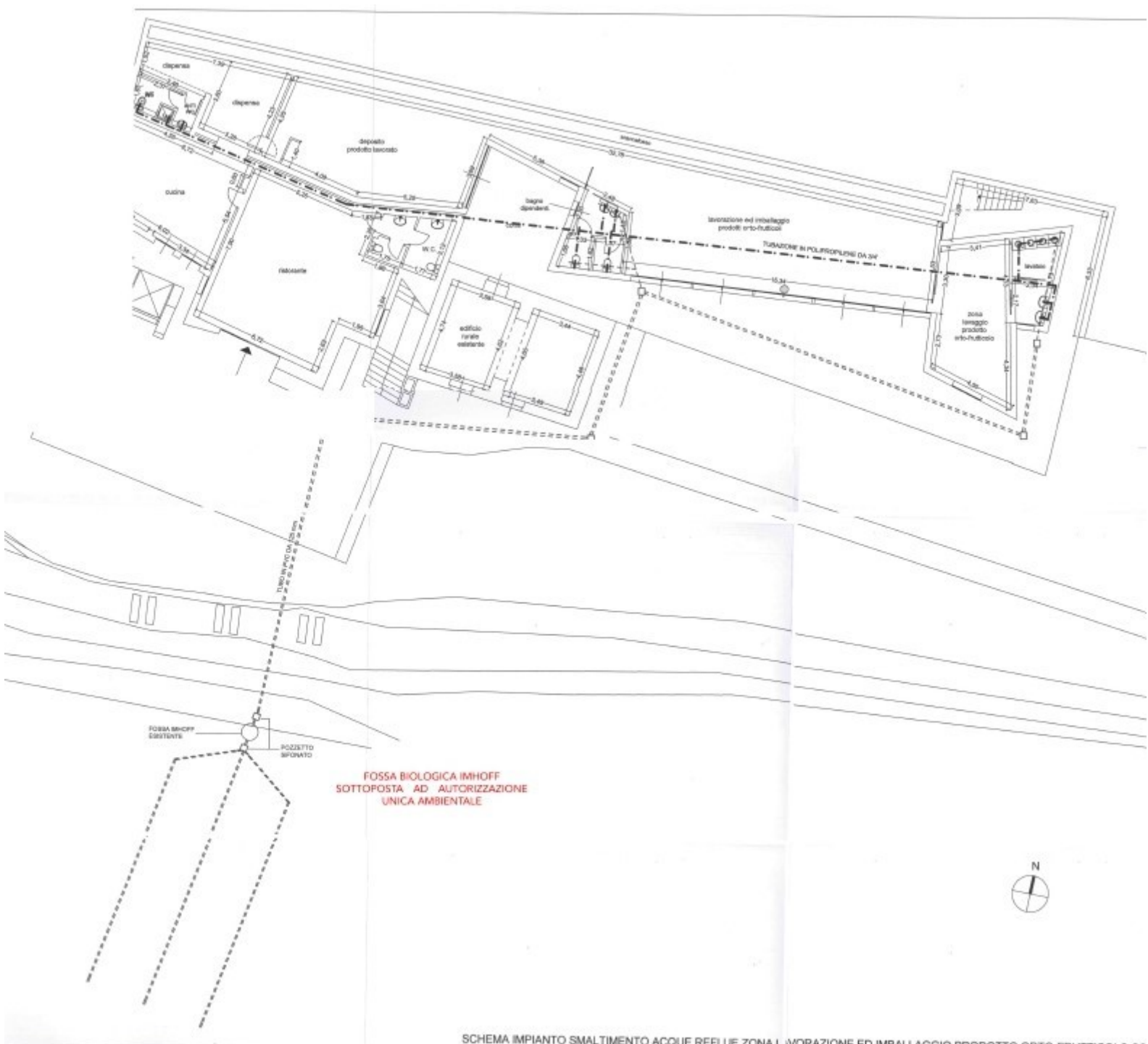
SCHEMA IMPIANTO SMALTIMENTO ACQUE REFLUE ZONA LAVORAZIONE ED IMBALLAGGIO PRODOTTO ORTOFRUTTICOLO SC
